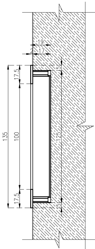
przekrój A-A
