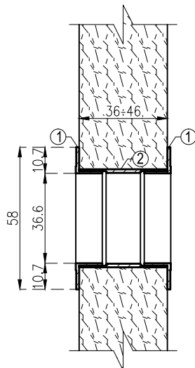
przekrój A-A
