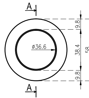
widok z tyłu (element 1)
