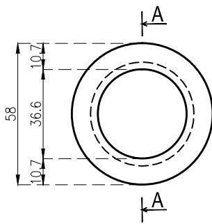
widok z przodu/z tyłu (element 2)
