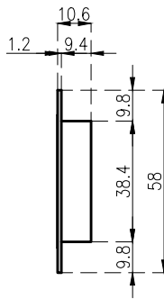
widok z boku (element 1)
