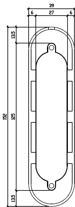
Widok z tyłu uchwyt I
