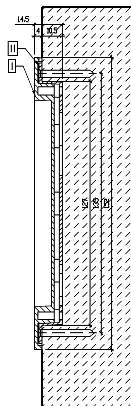
Przekrój A-A
