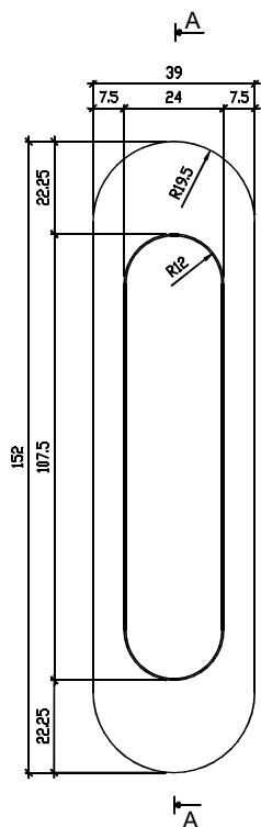
Widok z przodu uchwyt I
