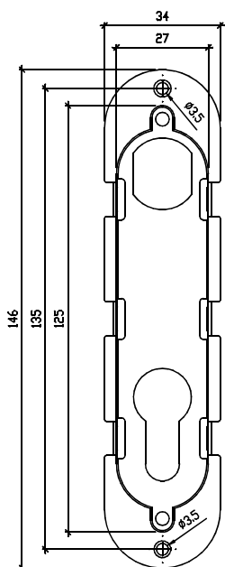
Widok z przodu rozeta montażowa II
