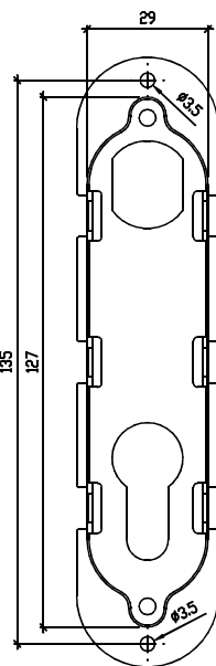
Widok z tyłu rozeta montażowa II
