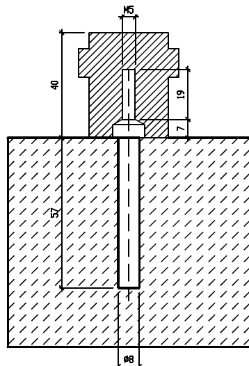
Przekrój A-A
