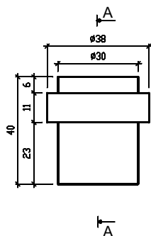
Widok z przodu odbój I
