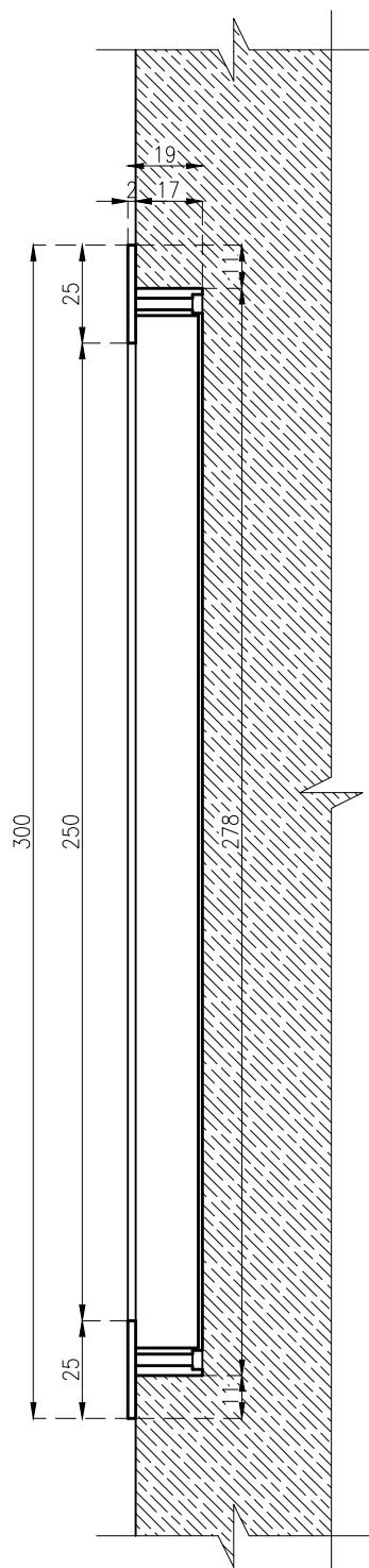
przekrój A-A
